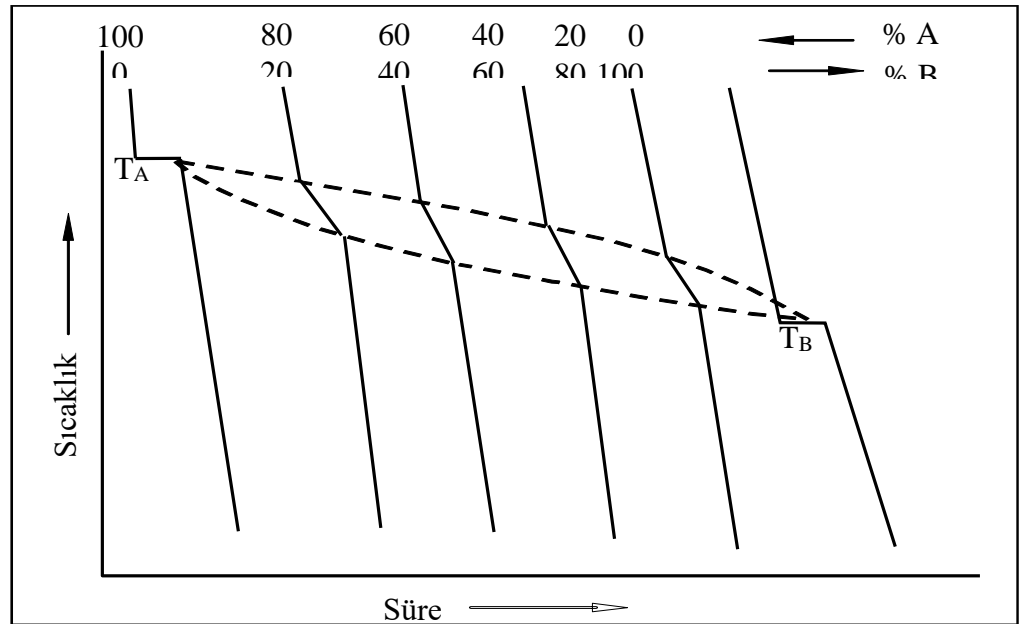
Şekil 2.2. Birbiri içerisinde her oranda çözünen iki metalin oluşturduğu sisteme ait alaşımların soğuma eğrileri.
